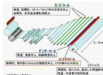
フィルム製造ラインへの実用例
