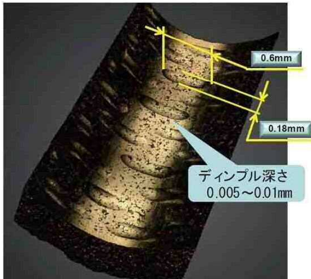
軸受内径拡大写真
